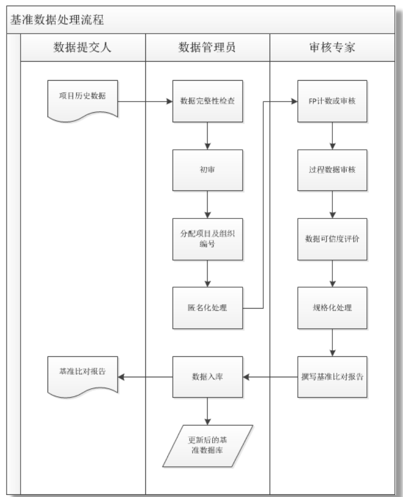
图 3.1 基准数据处理流程
