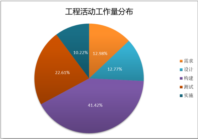
图 4.6 工作量分布
