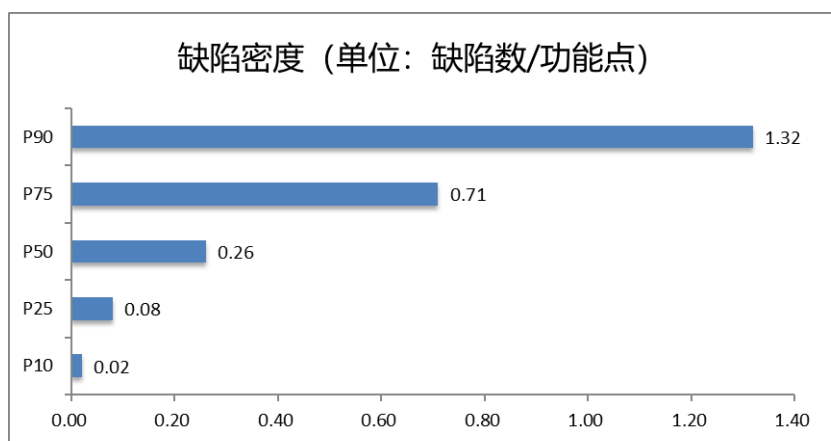
图 4.4 缺陷密度
