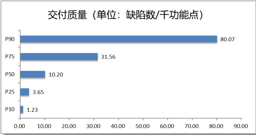
图 4.5 交付质量
